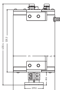
zijaaanzicht
