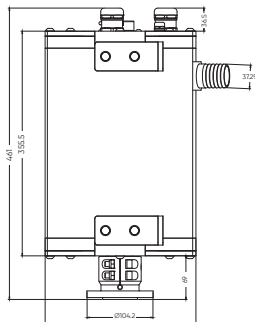
zijaaanzicht
